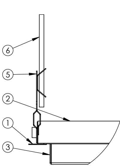
Montagem da estrutura
