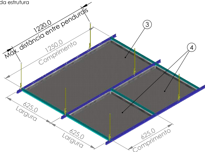
Isométrica da estrutura
