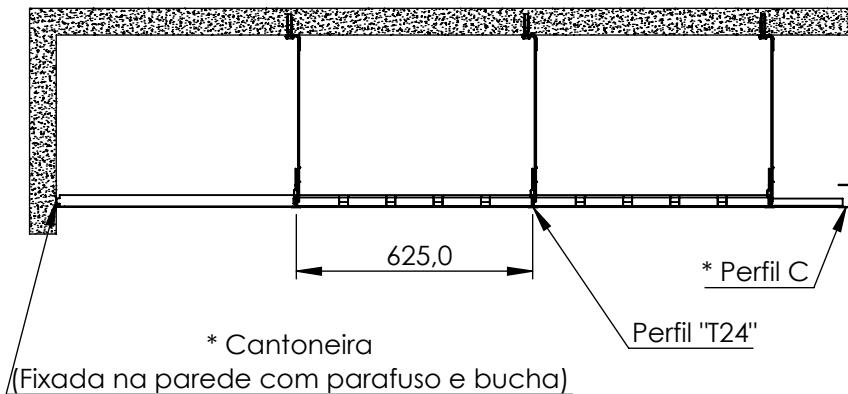
Fixação do Perfil "C"
