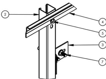
DETALHE A
