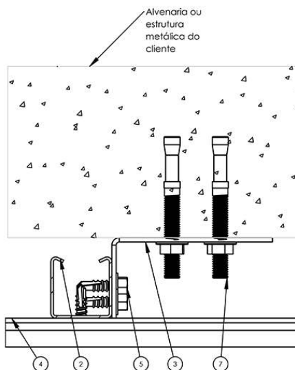
Fixação da estrutura ESCALA 1 : 2
