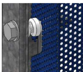
Ajuste rápido para espaçamento uniforme
