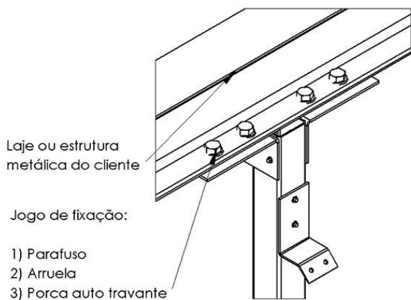
Fixação tipo 2: Perpendicular
