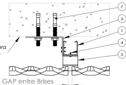
DETALHE B Fixação tipo 1: Paralela
