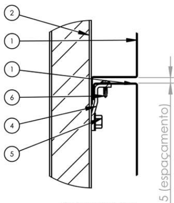
DETALHE Fixação das bandejas
